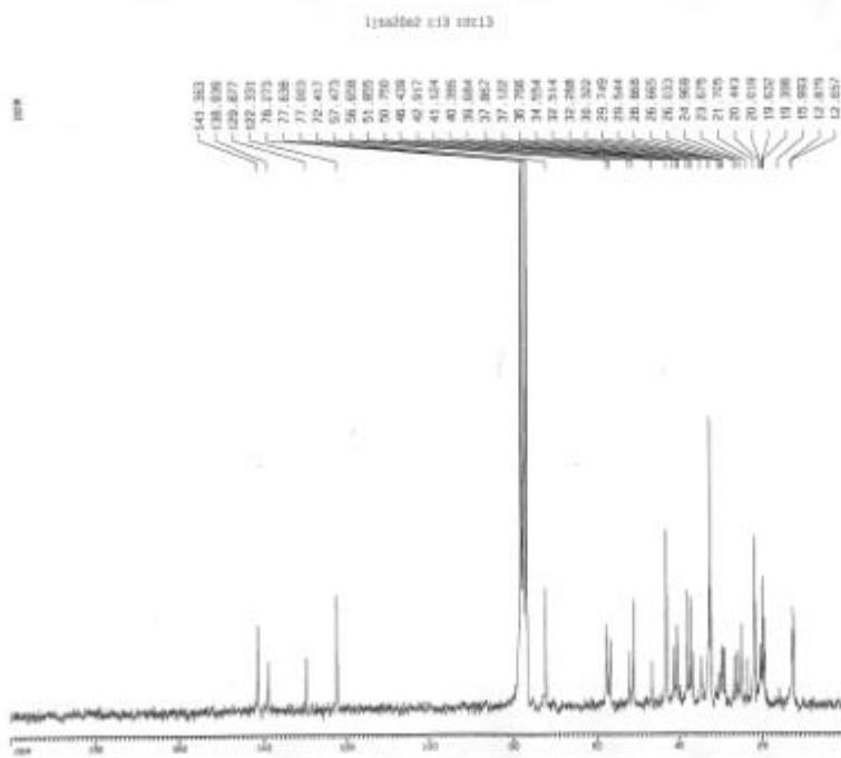
圖 13 : ^{13}\text{C} -NMR spectrum of compound IV
